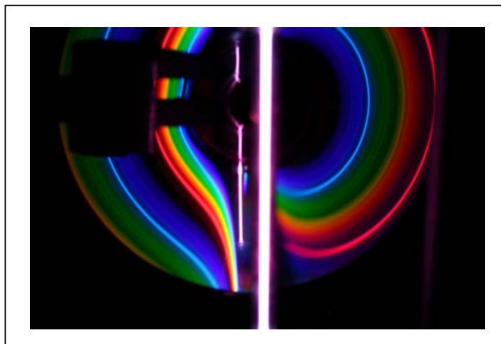
Spettro dell'Idrogeno fotografato grazie al riflesso di un CD
